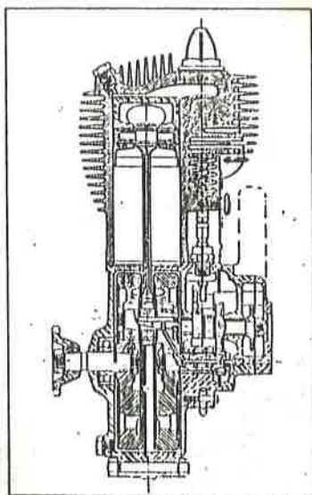
Moteur 350 Standard.
