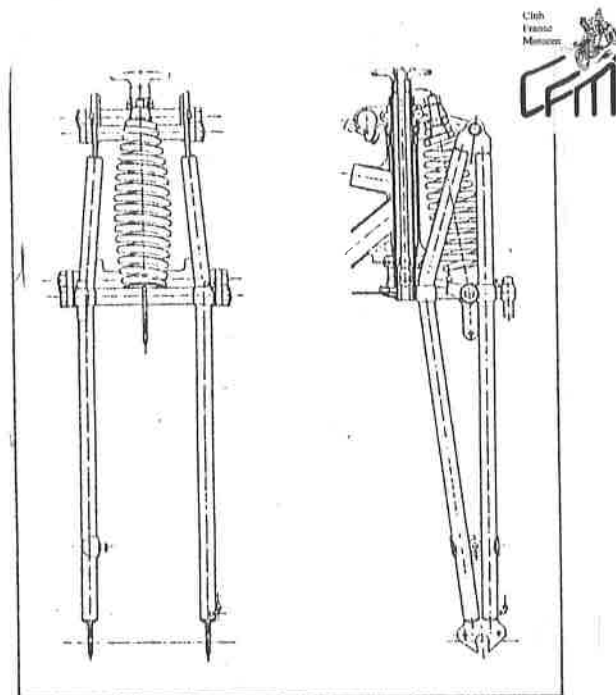
La fourche type « Webbs » de l'H.L.G. 1932.
