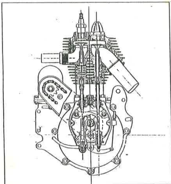
Moteur 350 Standard.
